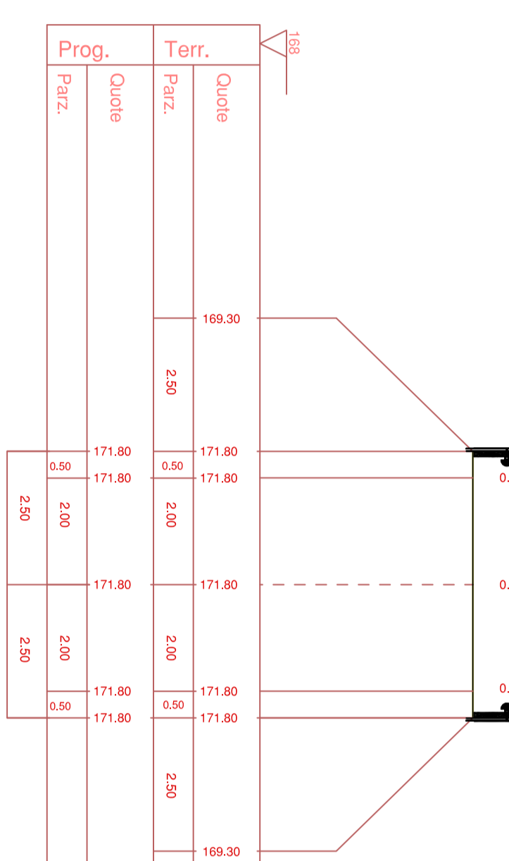
Sezione 11 Prog: 00000 Azione: 000 Amm: 000 Scala: 1:100
