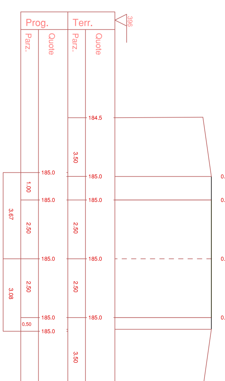
Sezione 3 Prog: 000 Azione: 000 Amm: 000 Scala: 1:100
