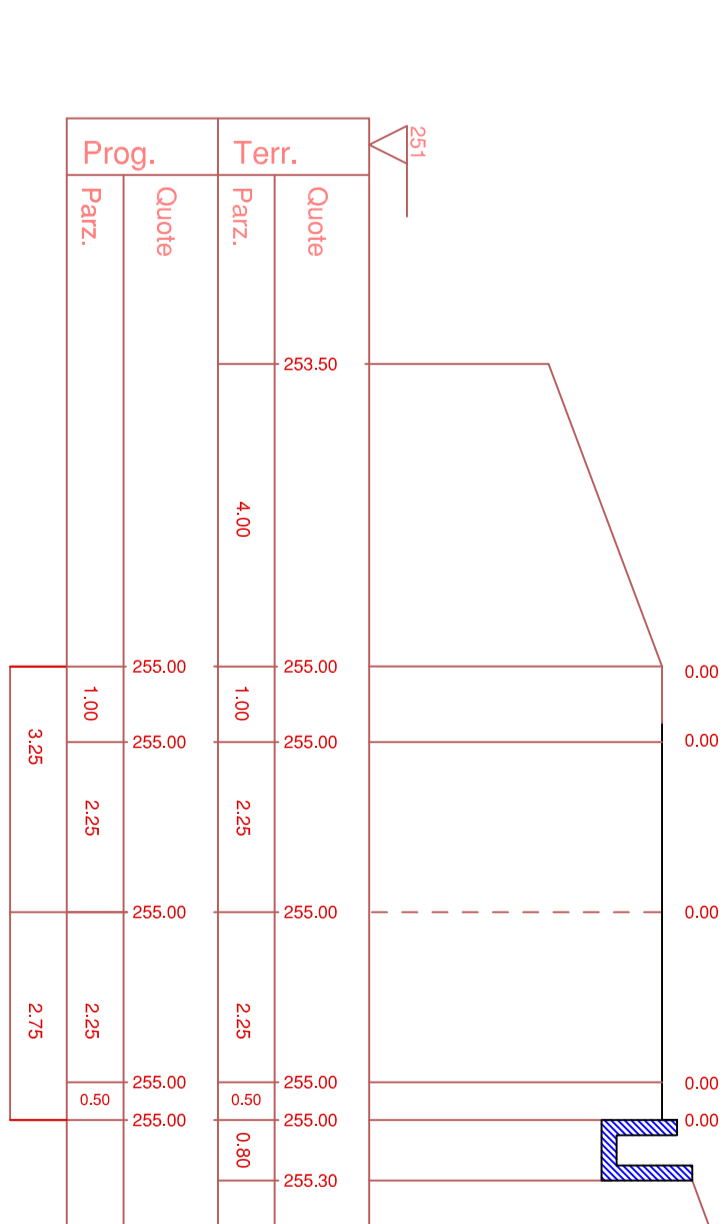
Sezione 31 Prog: 00000 Azione: 000 Amm: 000 Scala: 1:100
