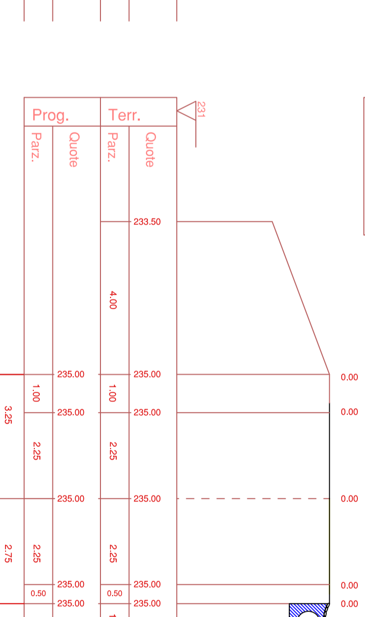
Sezione 24 Prog: 00024 Azione: 000 Amm: 000 Scala: 1:100
