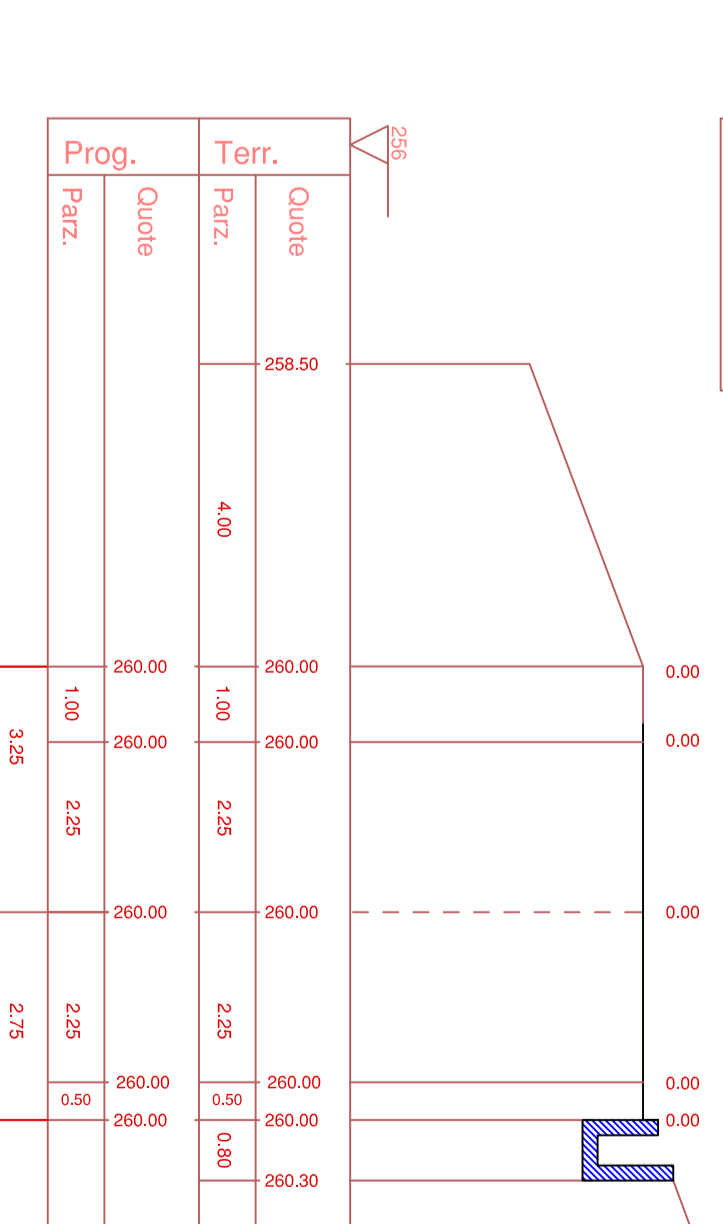
Sezione 32 Prog: 00032 Azione: 000 Amm: 000 Scala: 1:100
