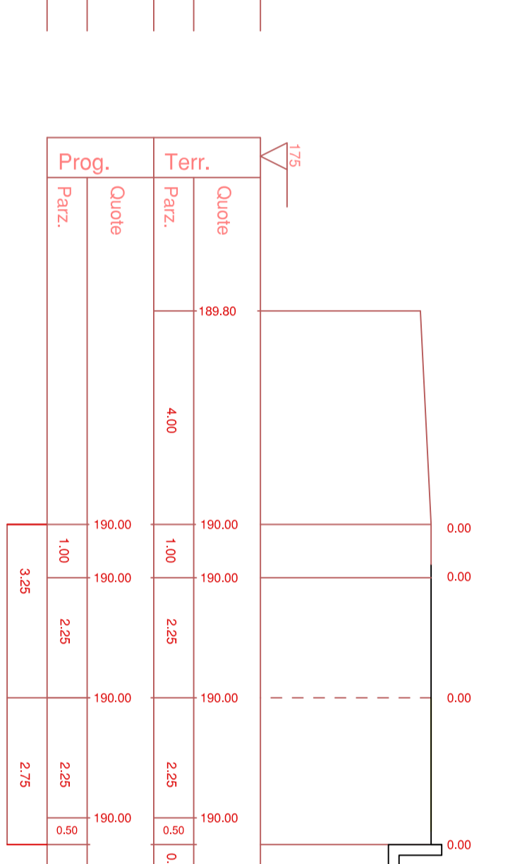
Sezione 15 Prog: 00000 Azione: 000 Amm: 000 Scala: 1:100
