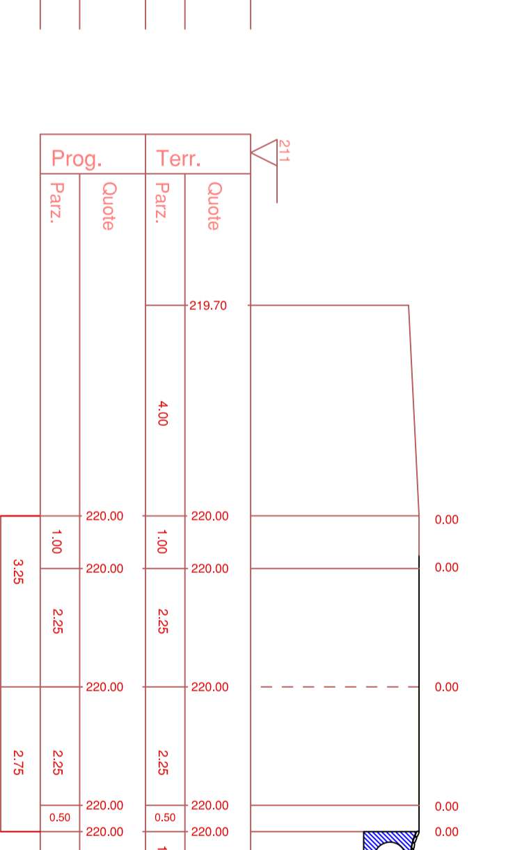
Sezione 21 Prog: 00000 Azione: 000 Amm: 000 Scala: 1:100
