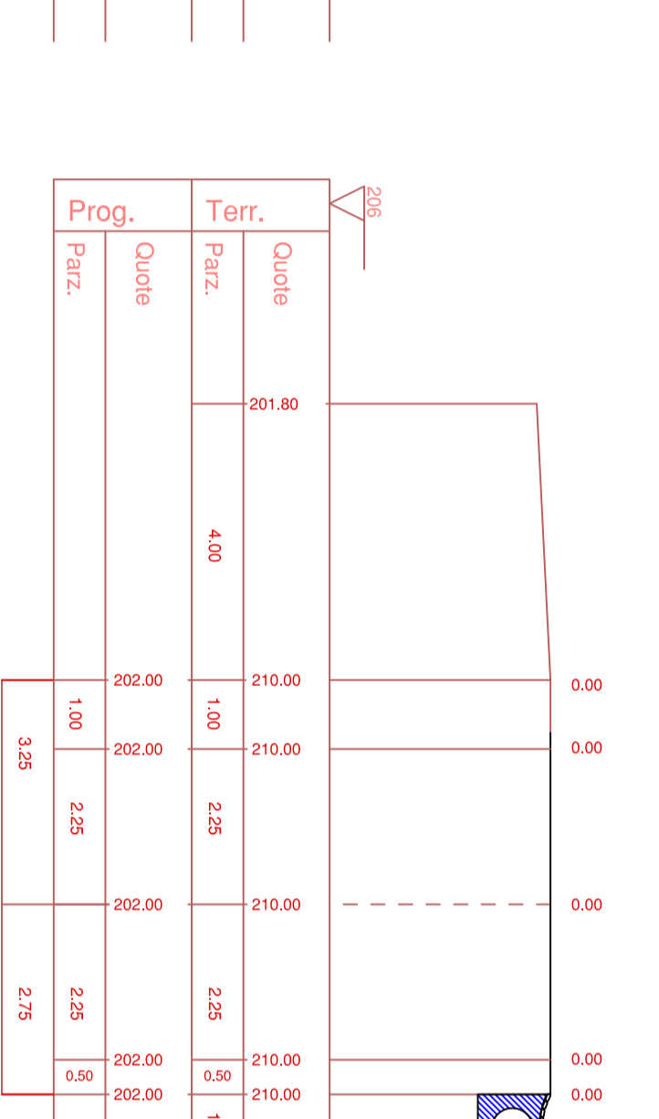
Sezione 17 Prog: 00000 Azione: 000 Amm: 000 Scala: 1:100
