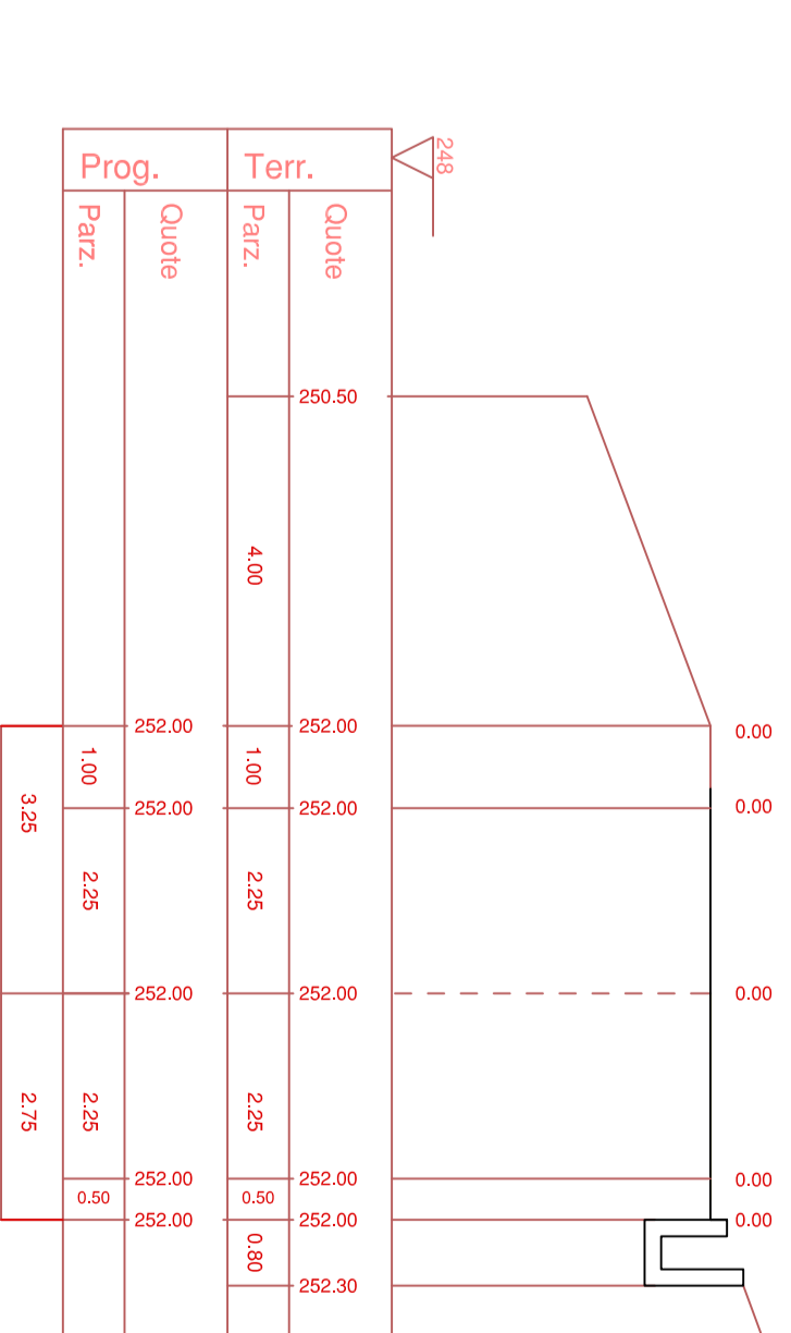
Sezione 29 Prog: 00000 Azione: 000 Amm: 000 Scala: 1:100
