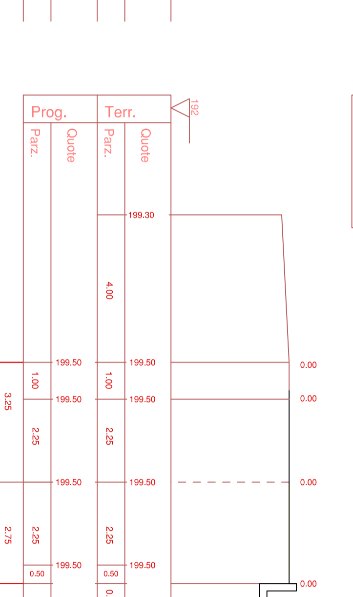
Sezione 16 Prog: 00016 Azione: 000 Amm: 000 Scala: 1:100
