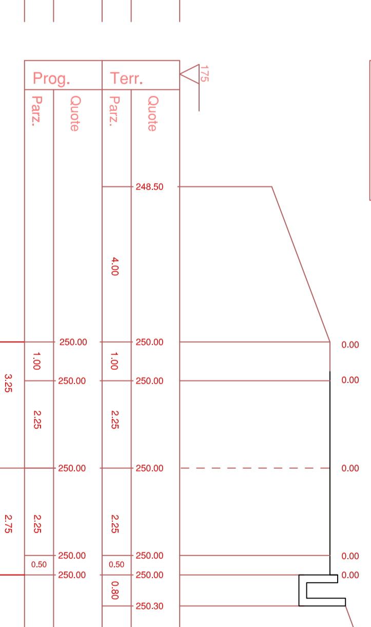
Sezione 28 Prog: 00028 Azione: 000 Amm: 000 Scala: 1:100
