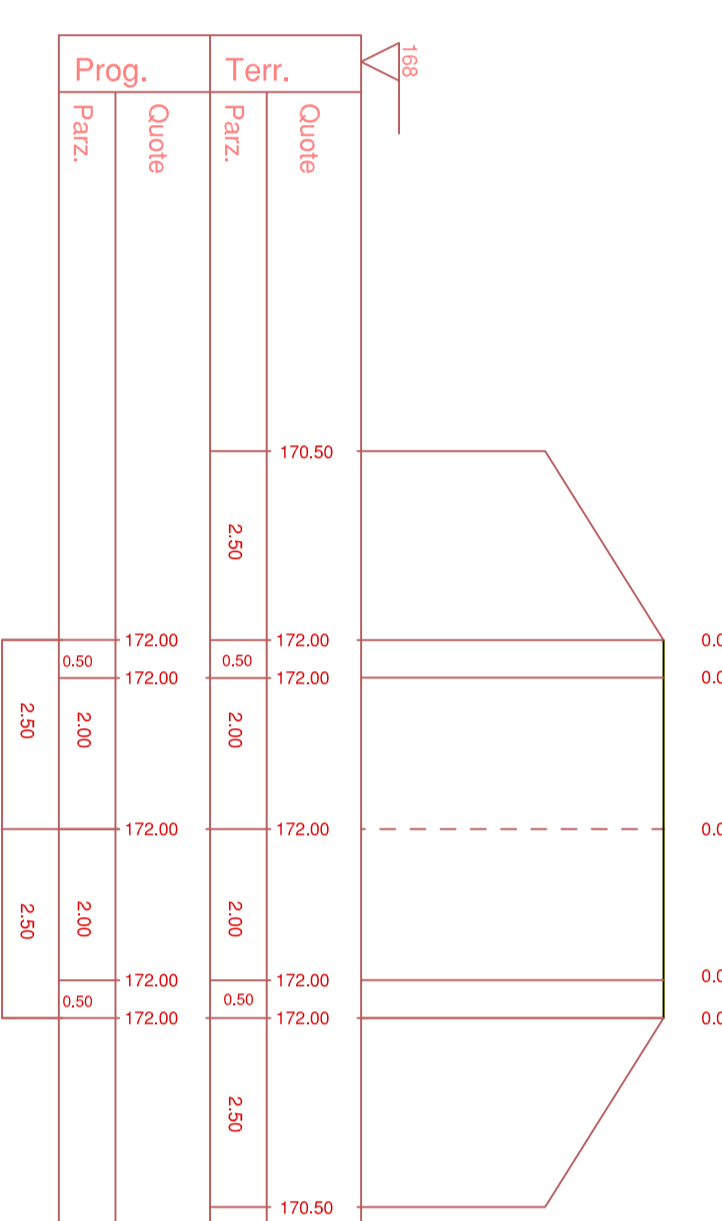
Sezione 9 Prog: 00000 Azione: 000 Amm: 000 Scala: 1:100
