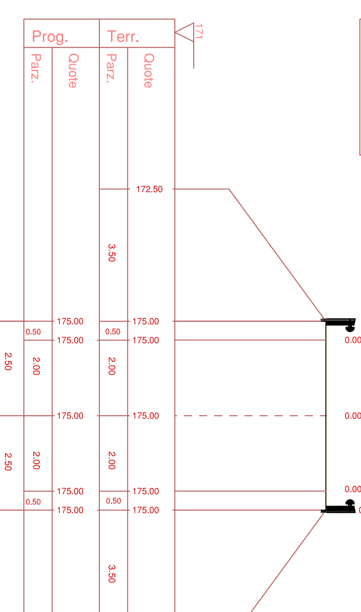
Sezione 4 Prog: 00004 Azione: 000 Amm: 000 Scala: 1:100
