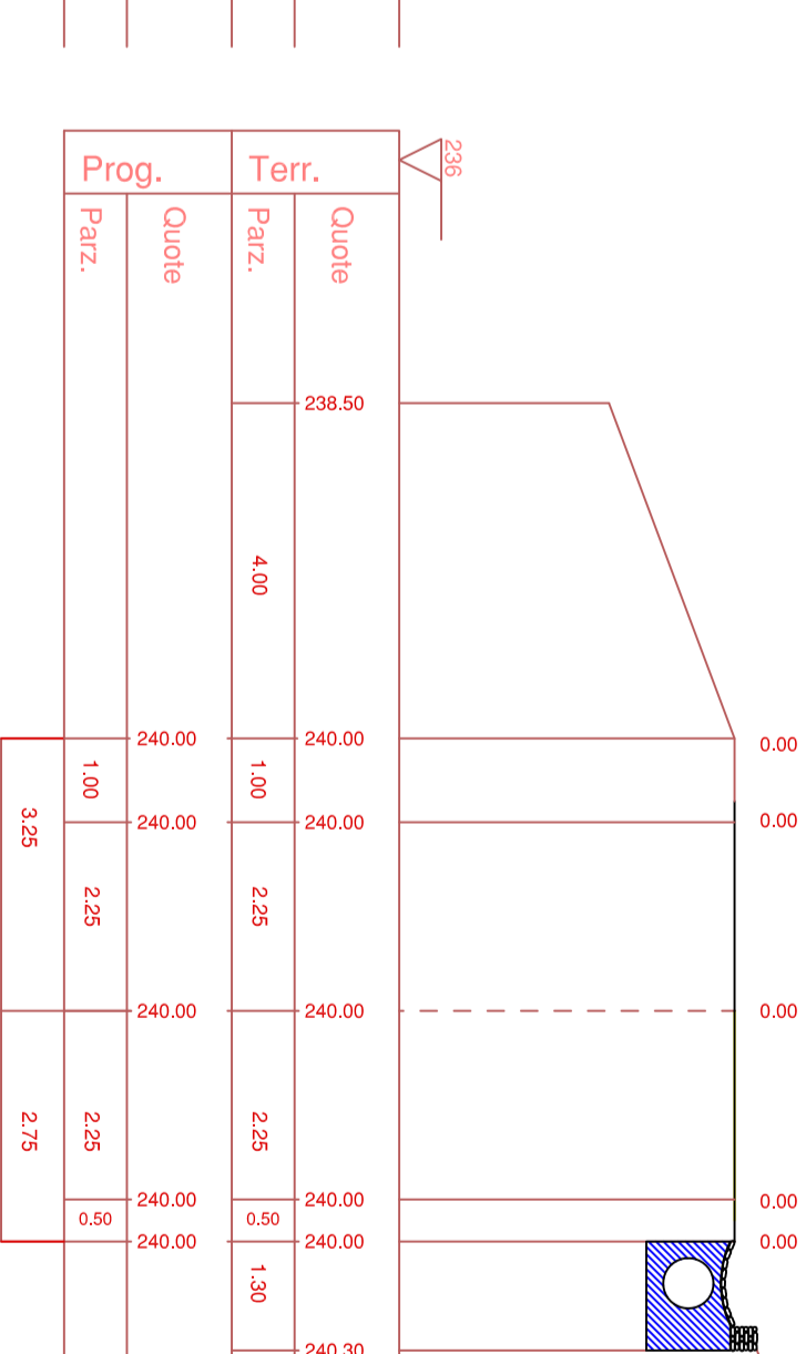
Sezione 25 Prog: 00000 Azione: 000 Amm: 000 Scala: 1:100
