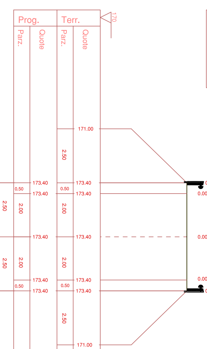
Sezione 8 Prog: 00008 Azione: 000 Amm: 000 Scala: 1:100
