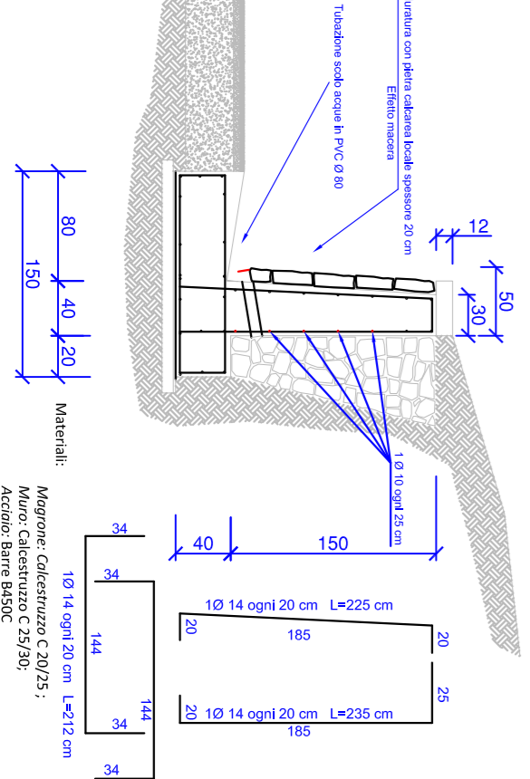
Muro tipo 3
