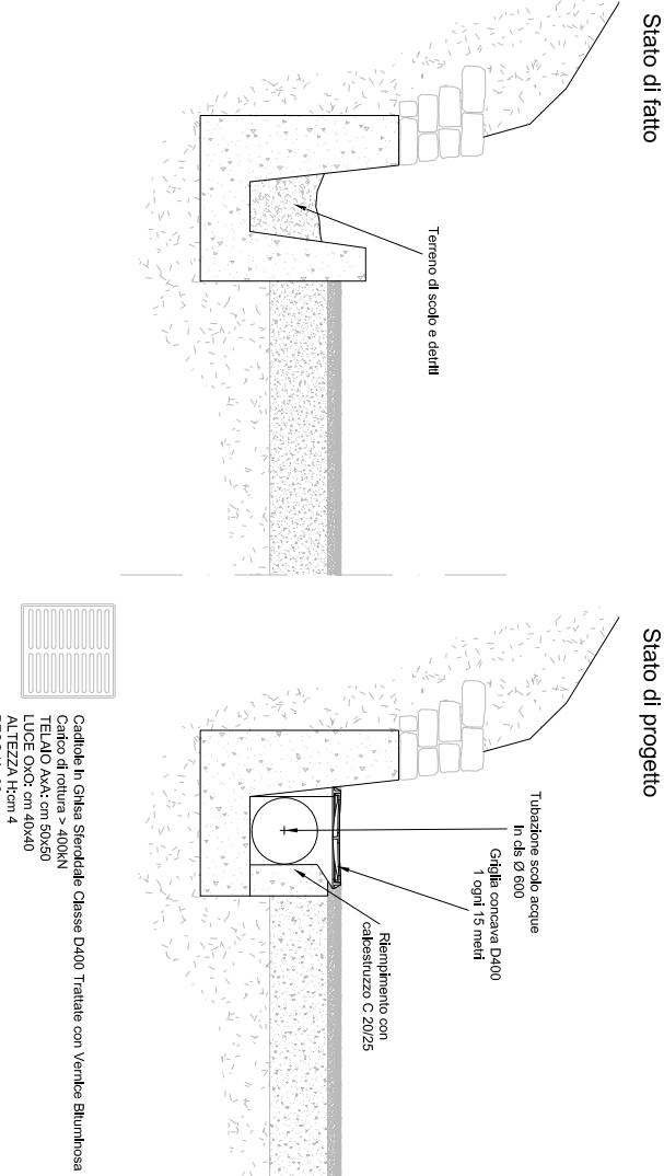
Cunetta Coperta
