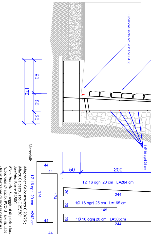
Muro tipo 4
